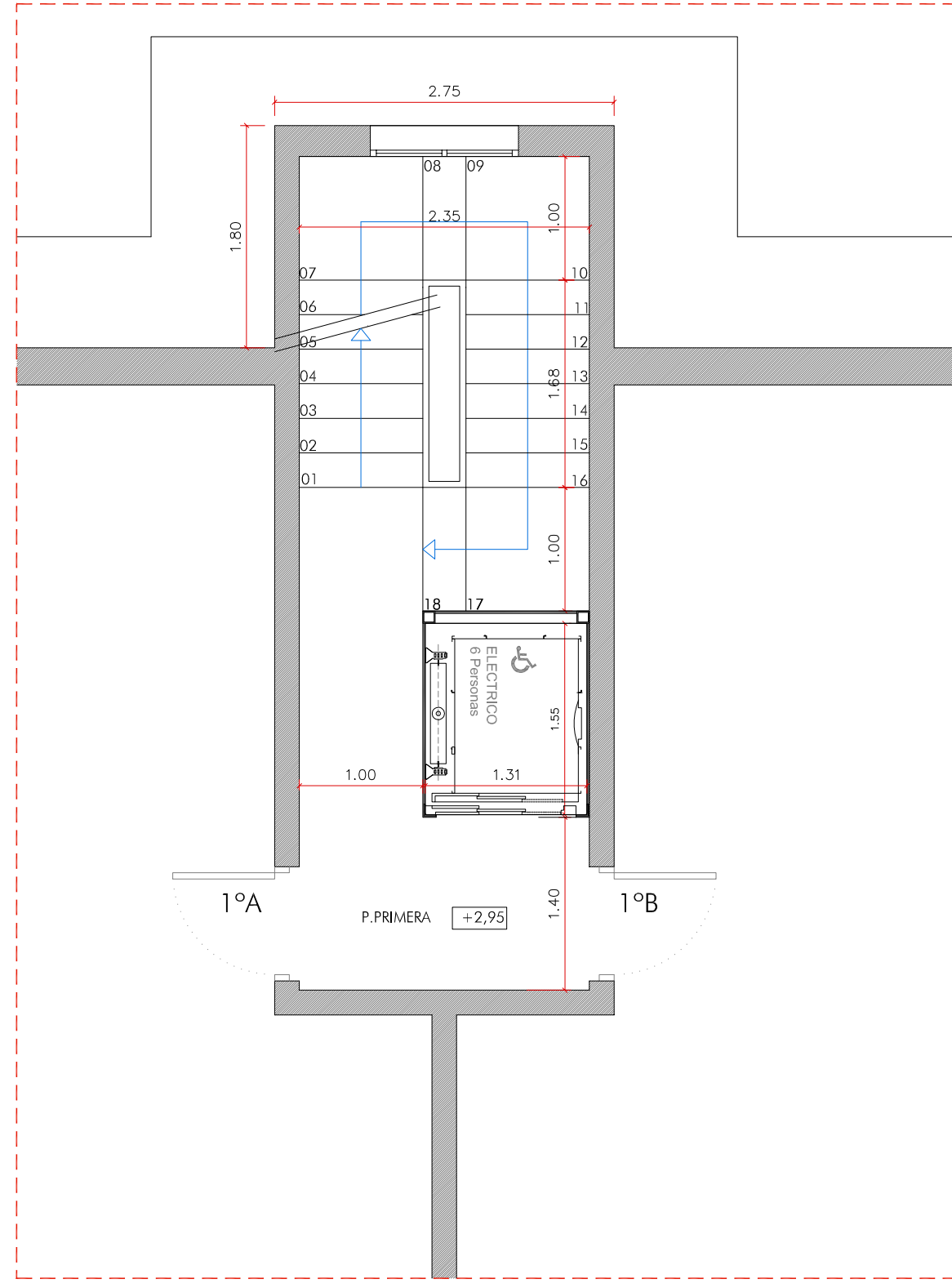
Planta Primera E 1:50
